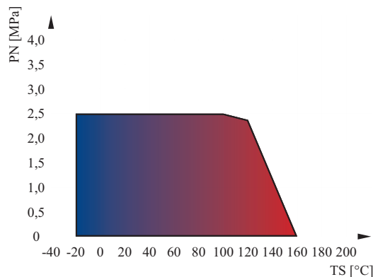
Wykres pola pracy kurka / Pressure-temperature diagram
